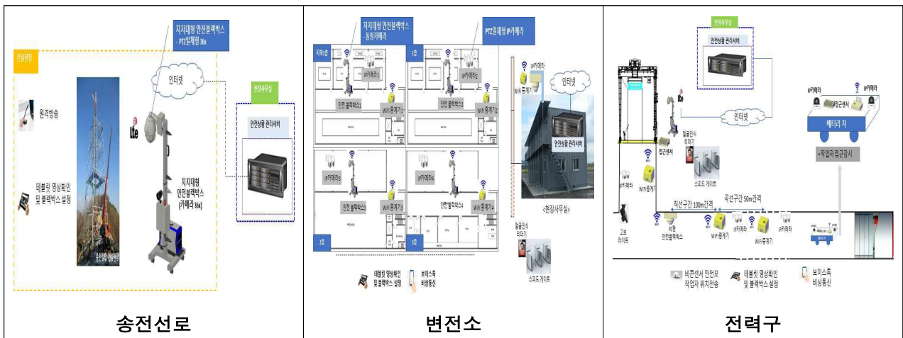
[그림 1] 스마트 안전블랙박스 건설현장별 모델
